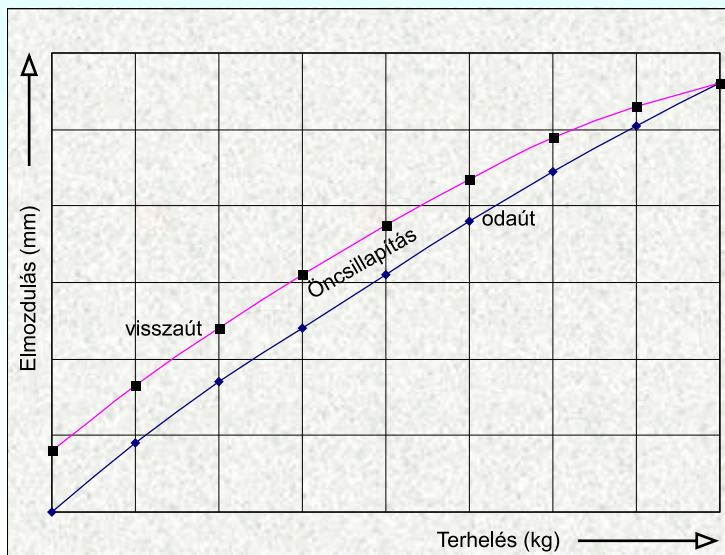
Rugózási diagramm
