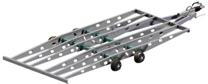
Alváz autószállító utánfutókhoz Teherbírási 3500 kg-ig
